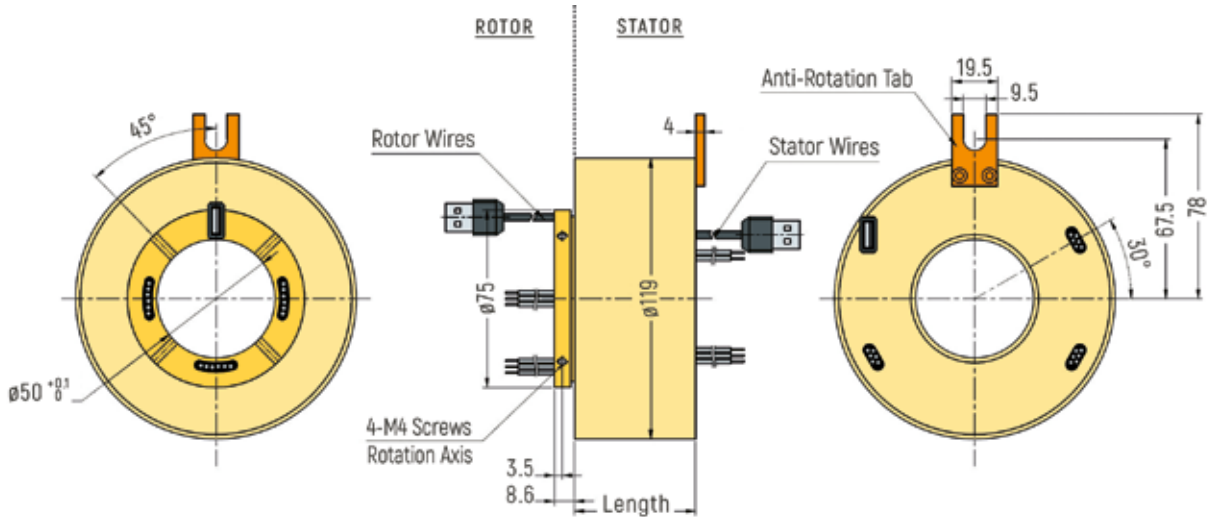
RX-USB501 - 1 USB Passage
