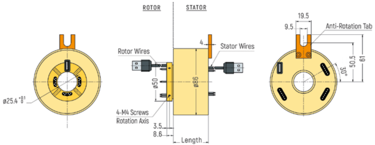
RX-USB251 - 1 USB Passage
