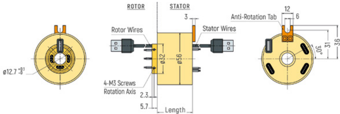
RX-USB121 - 1 USB Passage
