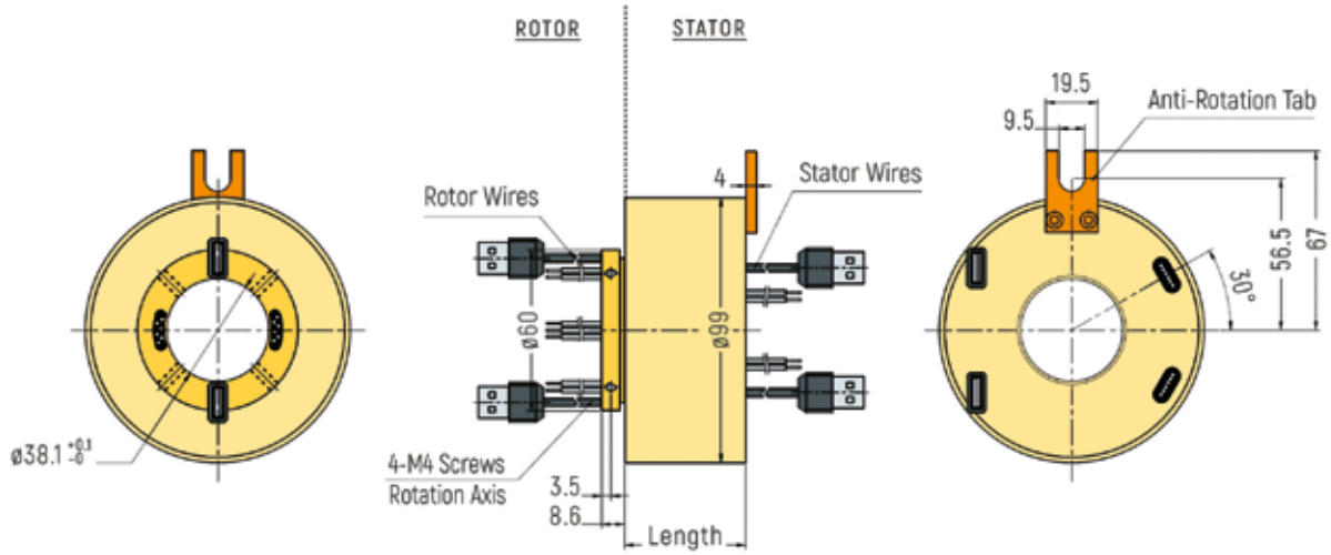
RX-USB382 - 2 USB Passages
