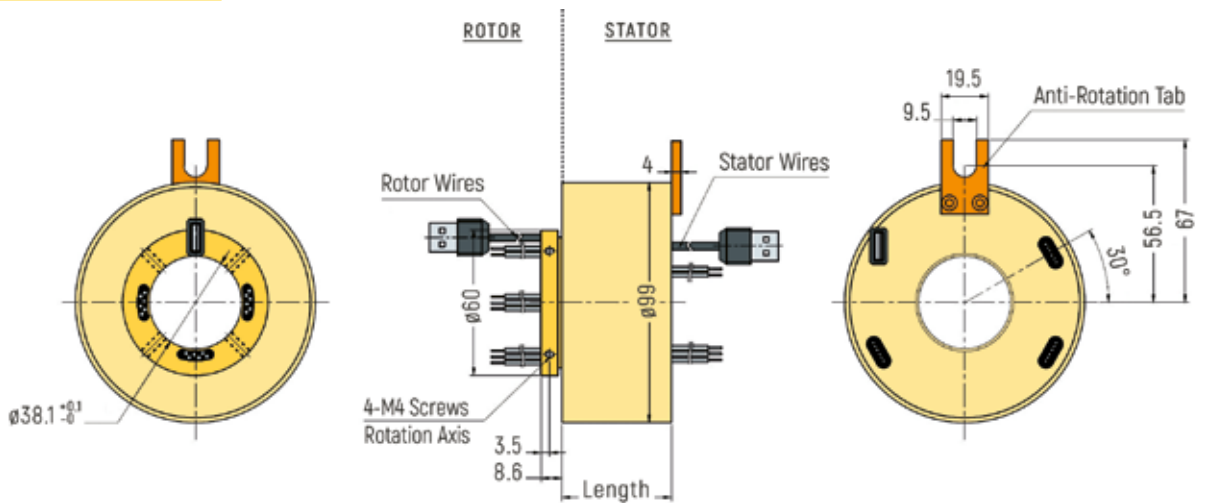
RX-USB381 - 1 USB Passage
