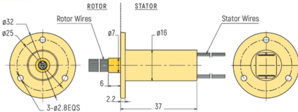
RX-MIN16D - 30 Rings / 2A
