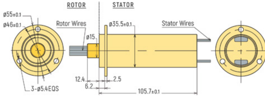
RX-MIN36A - 76 Rings / 2A
