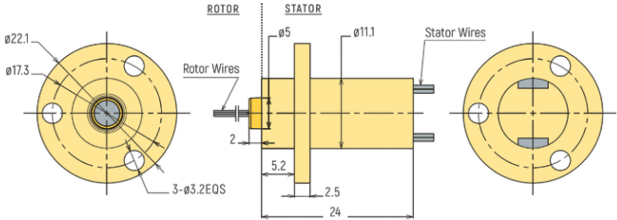
RX-MIN11B - 12 Rings / 1A
